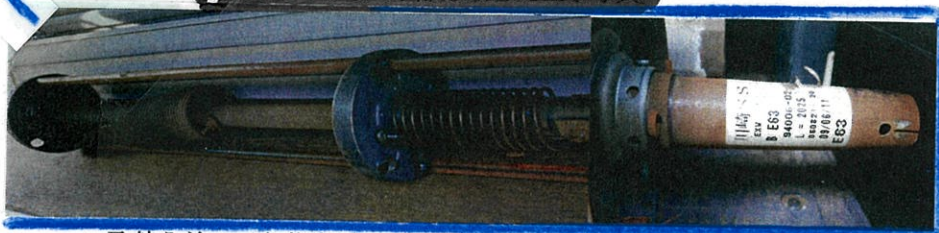
取替え前のバネ部分 (油切れ、ほこりまみれ、さび付き)
